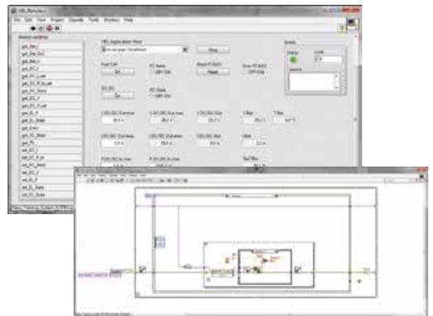
API-Erweiterungen
